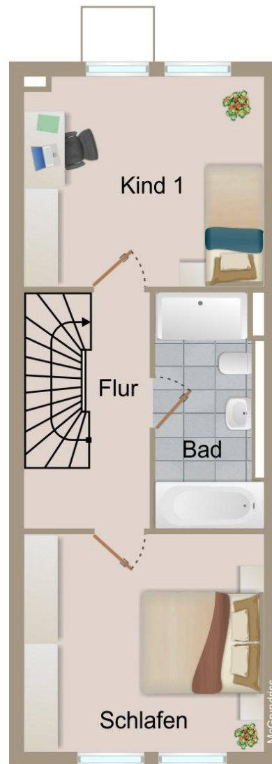
Grundriss Obergeschoss RMH 2, 3, 4
